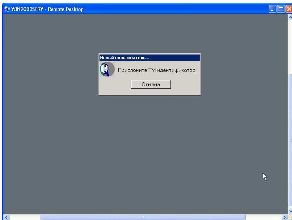
Рис. 25. Идентификация пользователя.
