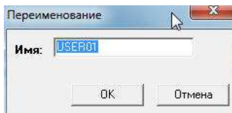
Рис. 8. Переименование пользователя
