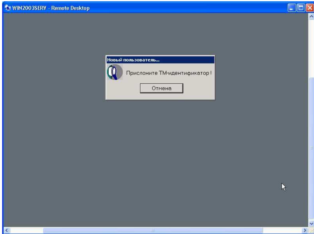
Рис. 25. Идентификация пользователя.
